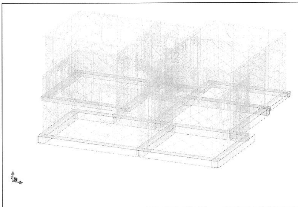
Figura 4 - Vista modello 3D con elementi in c.a. non verificati (IN GIALLO)
