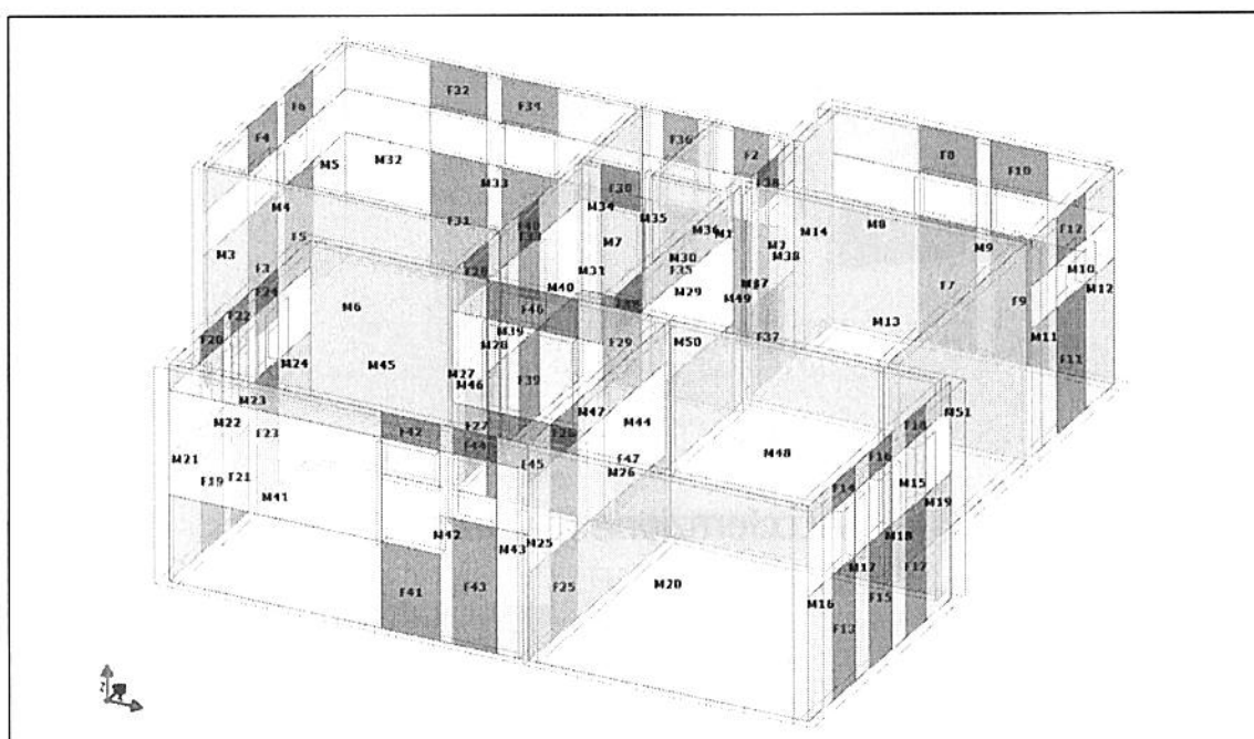
Figura 7 - Numerazione Maschi e Fasce murari al Piano Terra
